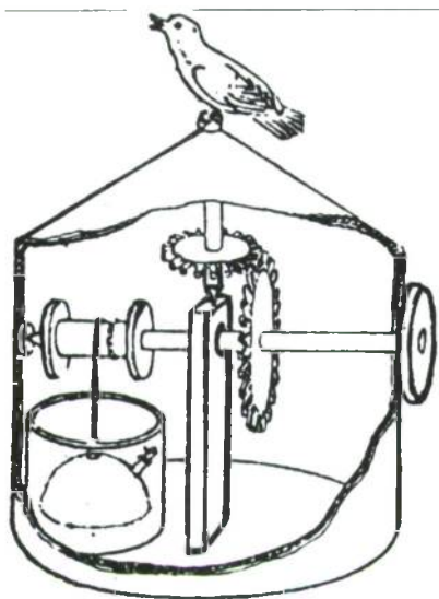
Η κατασκευή του Ήρωνα με οδοντωτούς τροχούς υπο γωνία, για τη μετάδοση κινήσεως.
