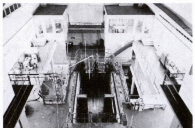
Εσωτερικό του κτιρίου του αντιδραστήρα. Διακρίνεται η δεξαμενή, ο θάλαμος ελέγχου και πειραματικές εγκαταστάσεις.
