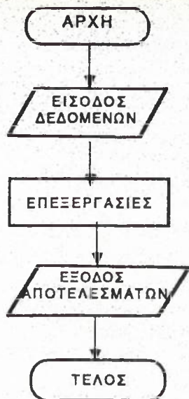
Δομή προγράμματος
